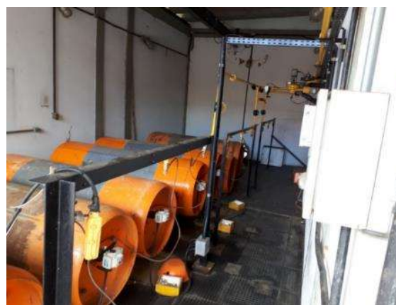
Figura 10 - Cilindros de 900 kg para o armazenamento do cloro gasoso
