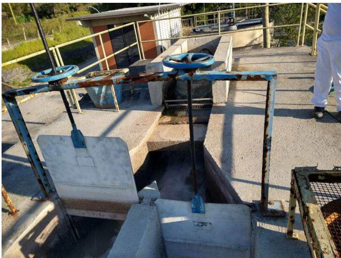
Figura 31 - Vista parcial do tratamento preliminar. Em primeiro plano comportas de entrada nas caixas de areia e ao fundo canal de chegada do esgoto bruto e gradeamento
