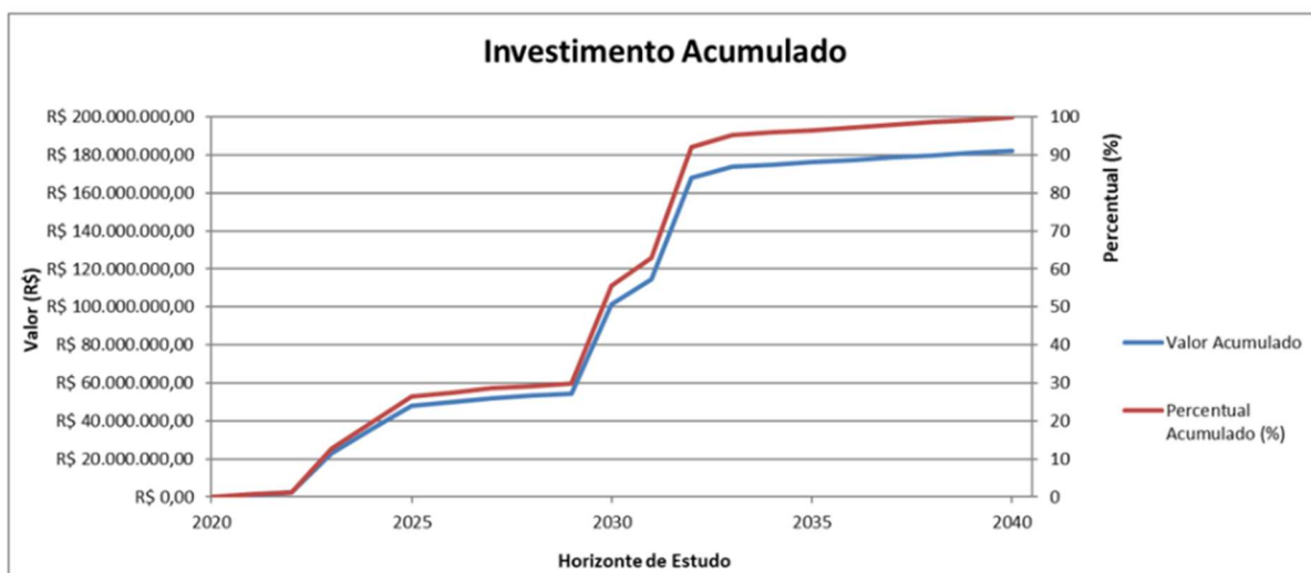
Figura 81 - Investimento acumulado no Sistema de Abastecimento de Água
